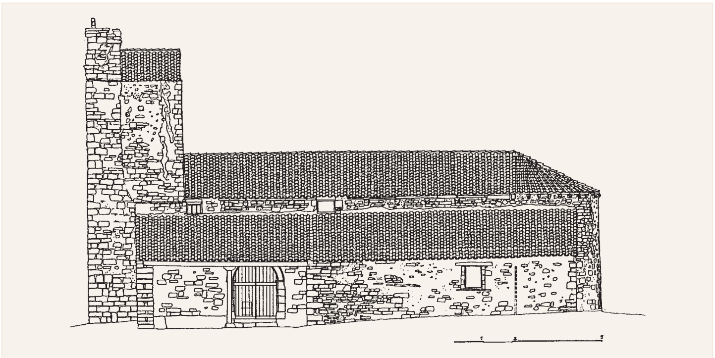
Alzado sur
