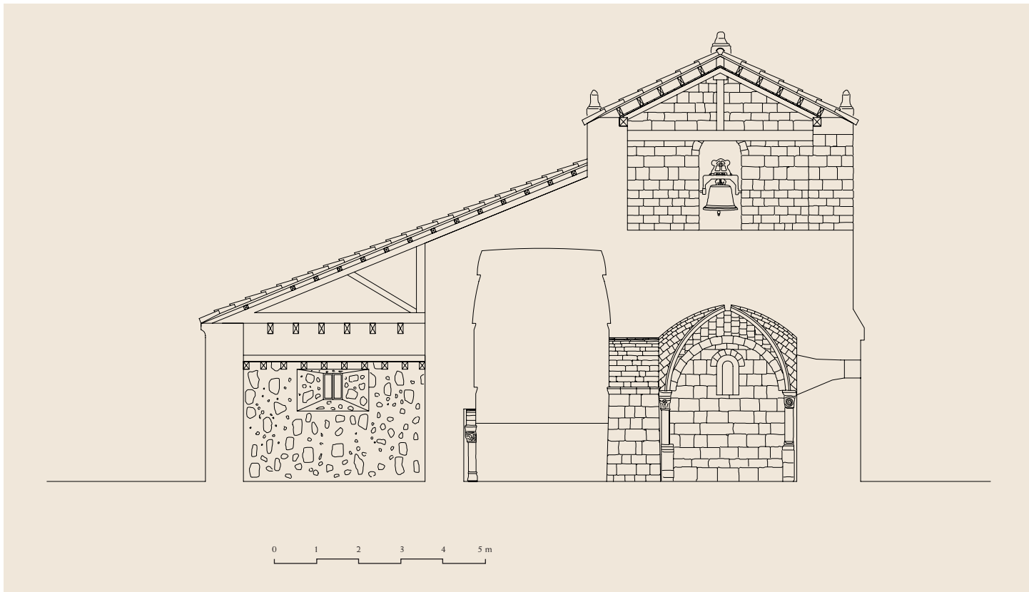
Sección transversal, por la torre
