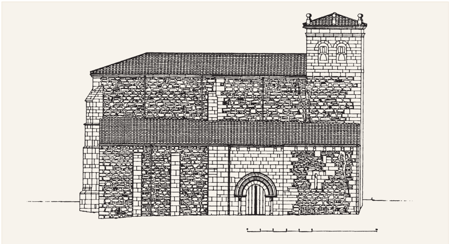
Alzado norte
