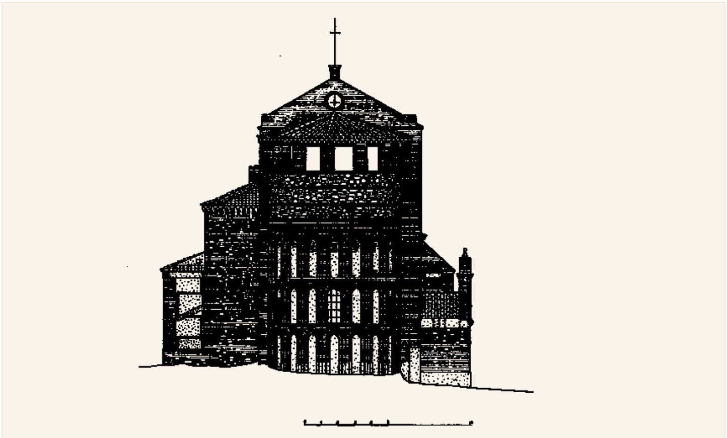
Alzado este
