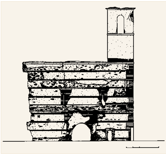
Alzado norte
