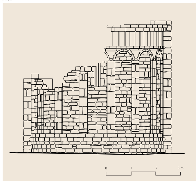
Alzado este
