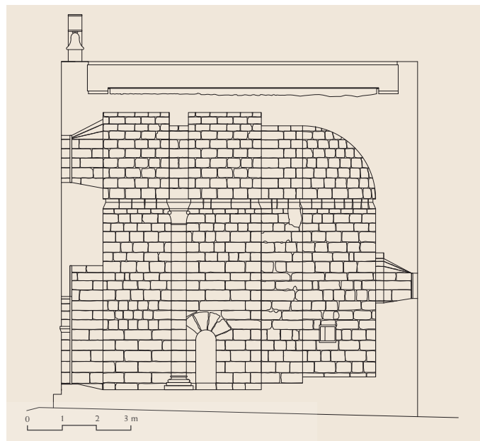
Sección longitudinal
