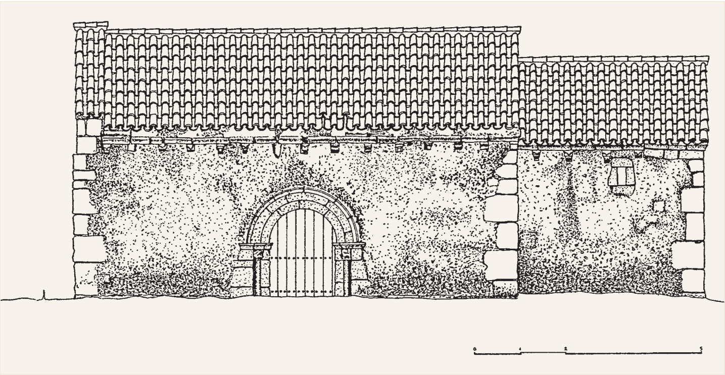
Alzado sur
