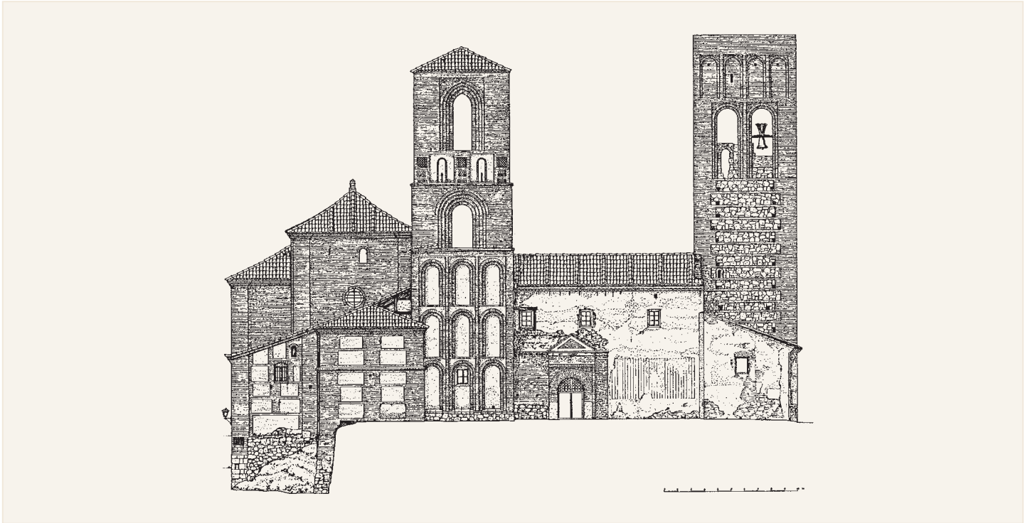
Alzado norte
