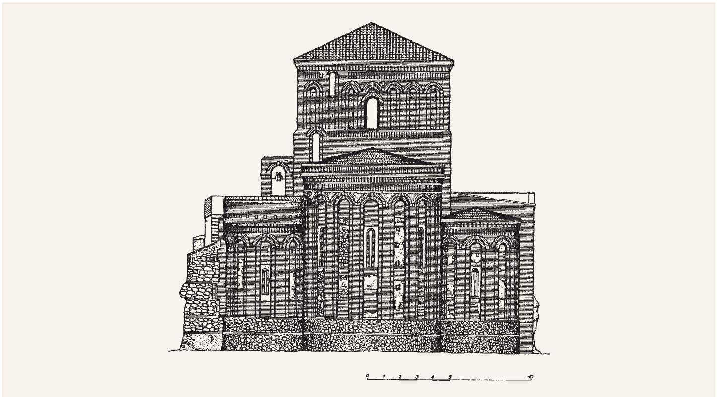
Alzado este
