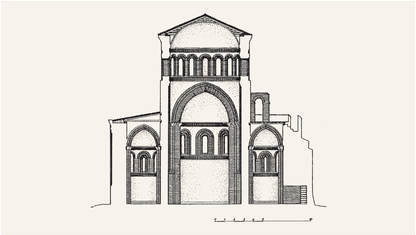
Sección transversal
