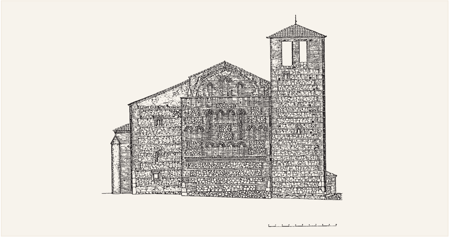
Alzado este
