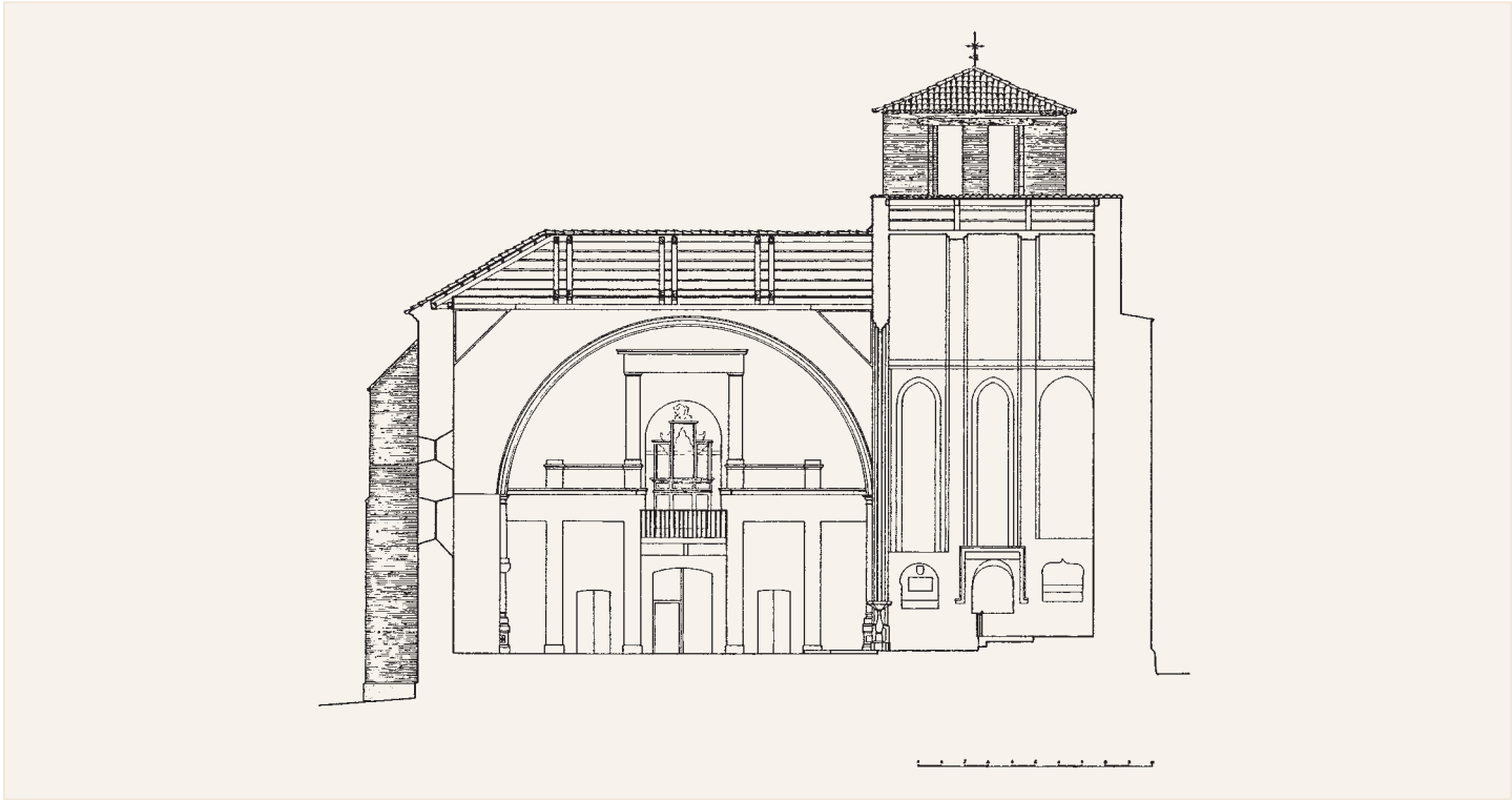
Sección longitudinal
